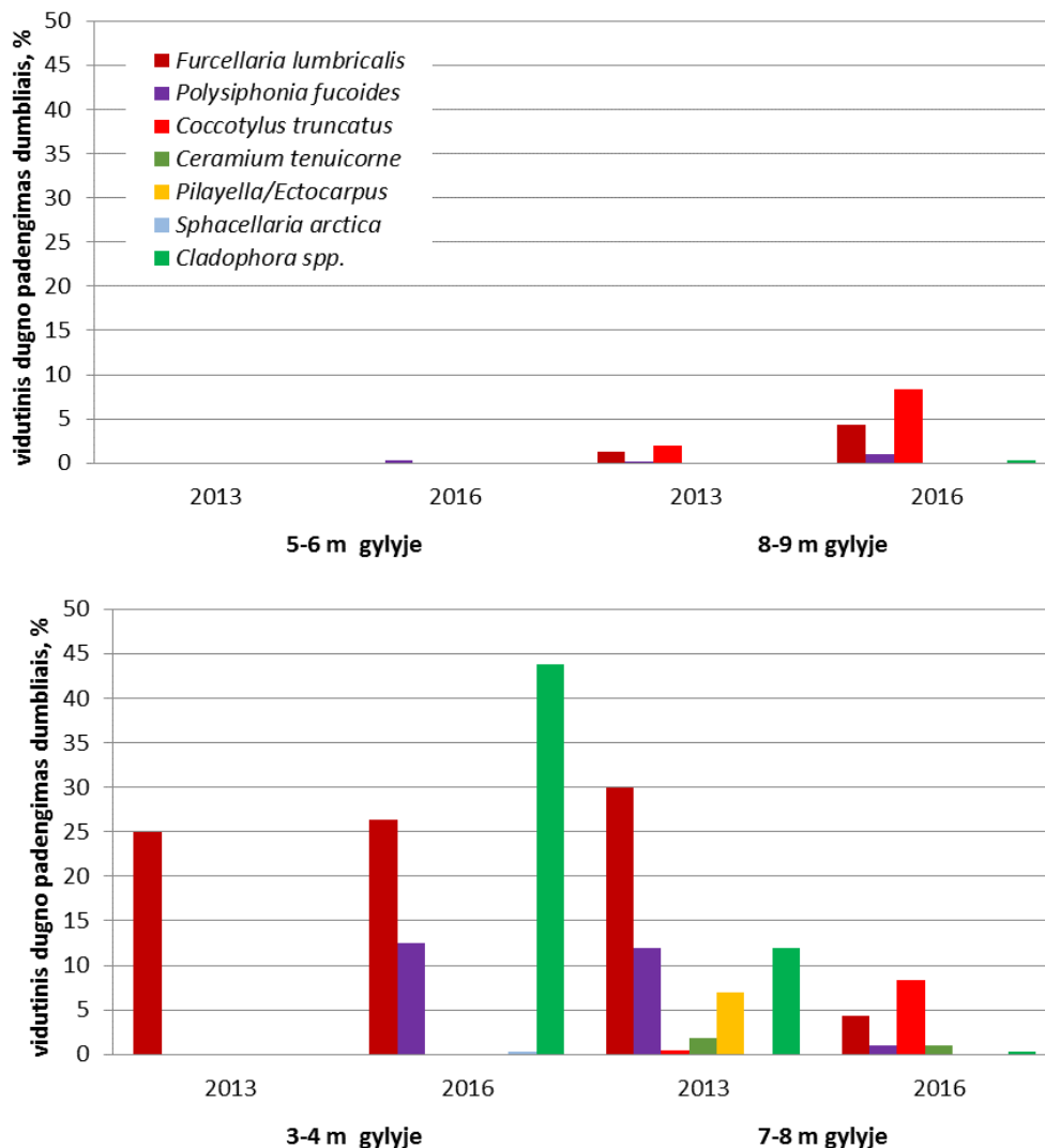
4 paveikslas. Lietuvos Baltijos jūros tarpinių vandenų (viršuje) ir priekrantės vandenų (apačioje) makrofitobentosos vidutinis gausumas (dugno projekcinis padengimas dumbliais) skirtinguose gyliuose 2013 ir 2016 m.
