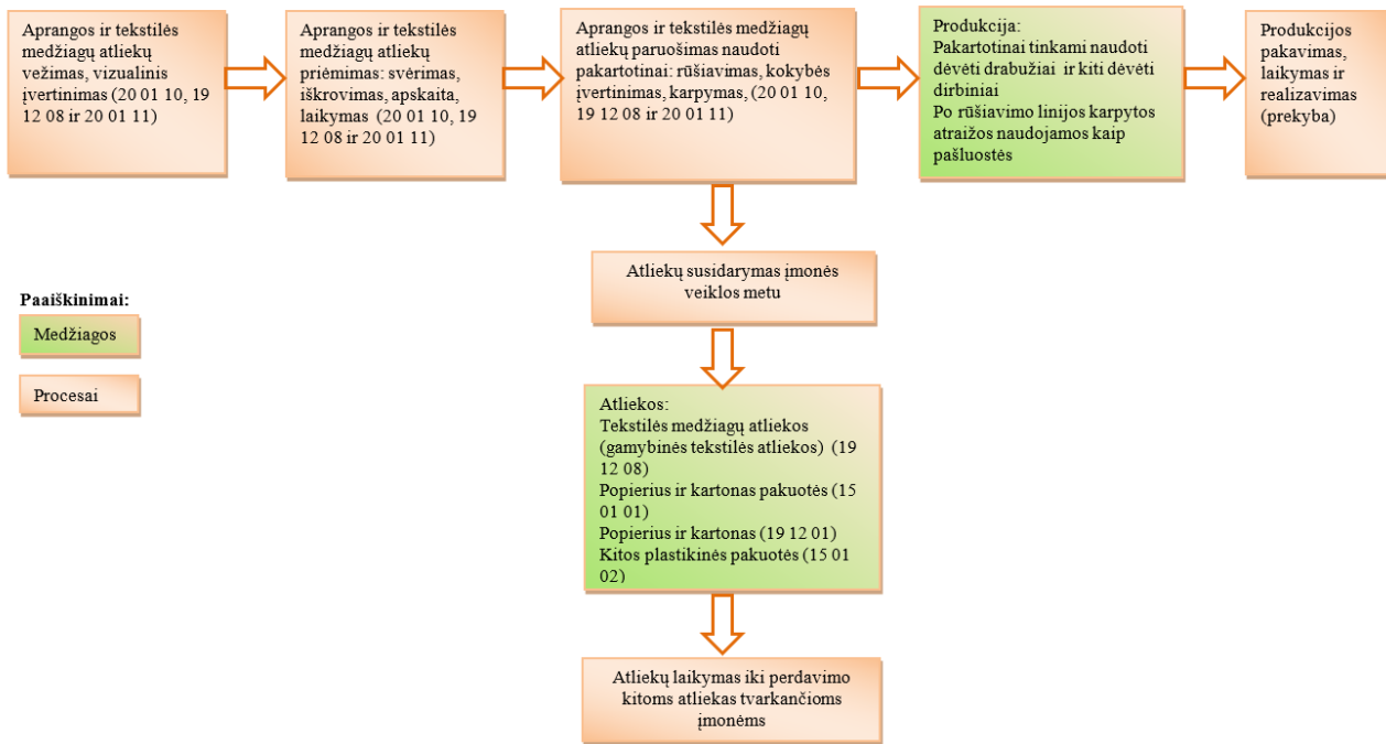
1 pav. UAB „Sentauras“ aprangos (atliekos kodas 20 01 10) ir tekstilės medžiagų (atliekų kodai 19 12 08 ir 20 01 11) atliekų tvarkymo technologinio proceso schema
