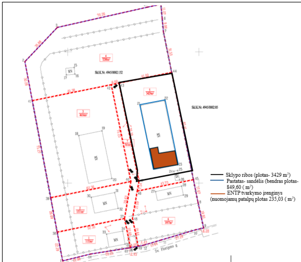
1 pav. UAB "Ožys" ENTP tvarkymo įrenginio išdėstymo teritorijoje planas
