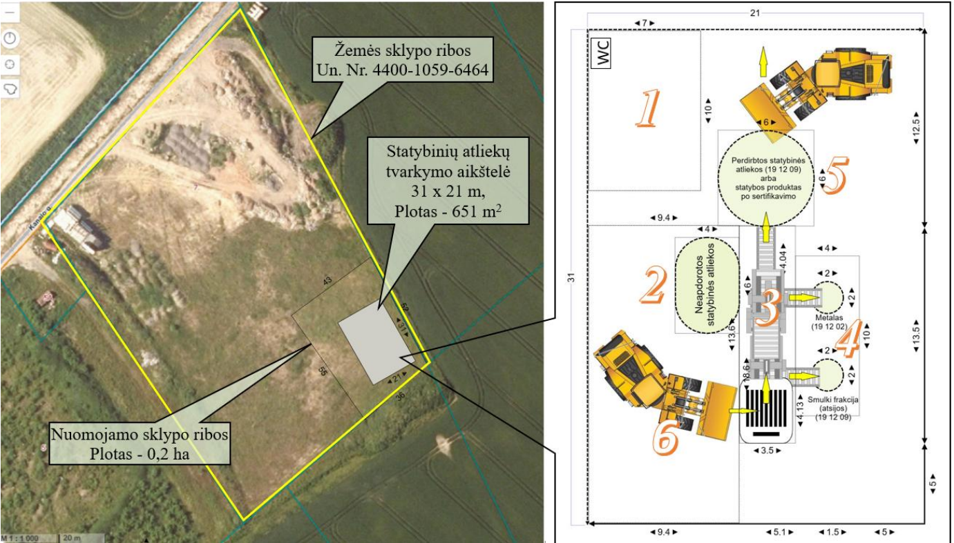
Veiklavietės funkcinį zonų išdėstymo planas
