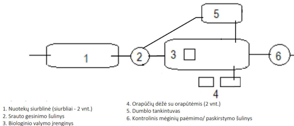
Pav. 2. . Technologinė valymo įrenginių schema
