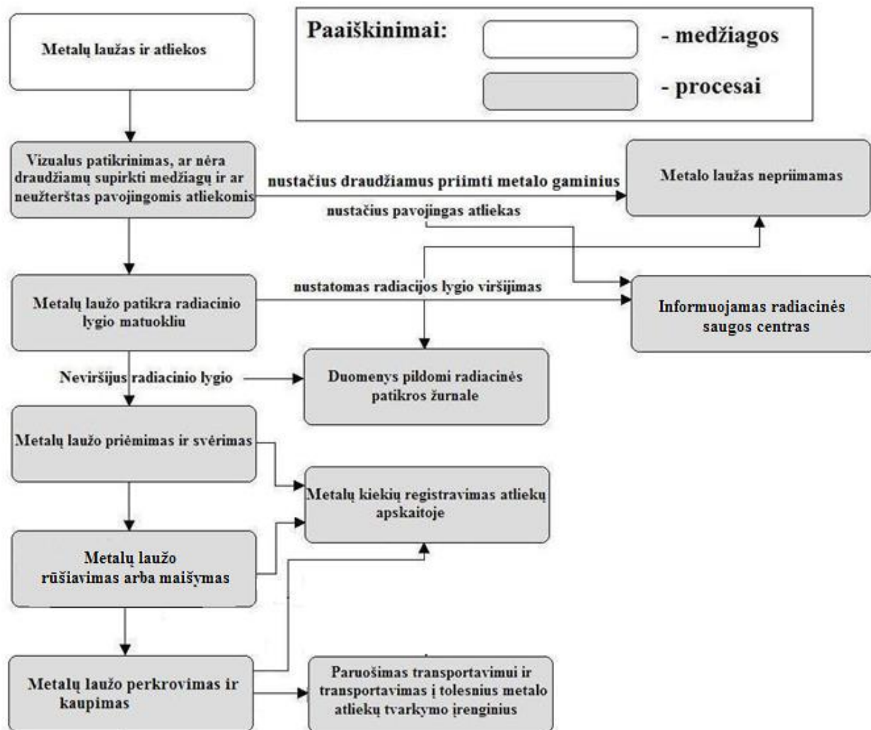
Netauriųjų metalų laužo ir atliekų tvarkymo technologinio proceso schema
